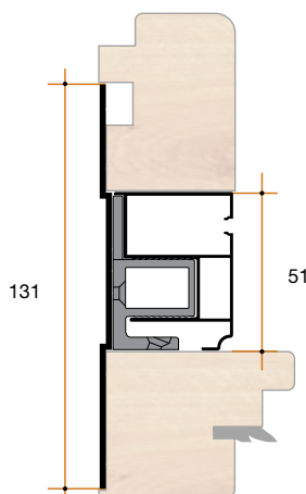
Esempio con guida e compensatore
