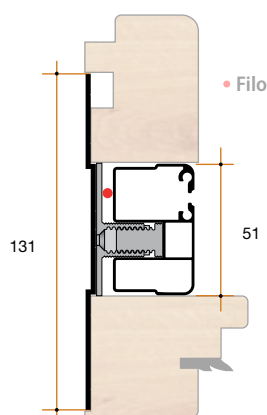
Esempio con guida e compensatore basso
