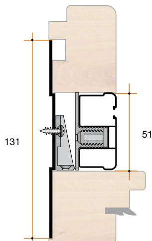
Esempio con guida e compensatore alto
