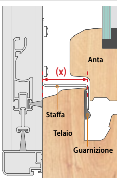
Serramento non complanare
