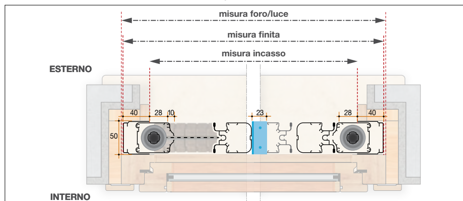
Sezione orizzontale 2 battenti con staffa attacco superiore con incasso 3 lati
