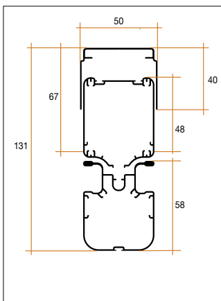
Ingombro cassa facile, cassonetto e barra maniglia
