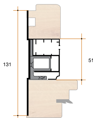
Esempio con guida e compensatore
