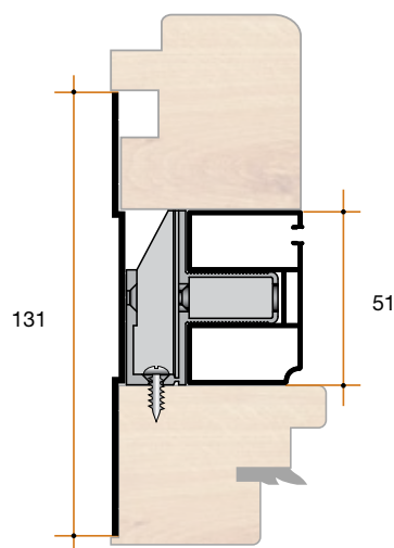
Esempio con compensatore alto.
