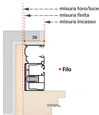
Esempio di installazione Guida Tapparella da 90 mm e compensatore basso
