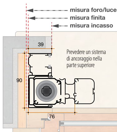
Esempio di installazione Guida Tapparella da 90 mm
