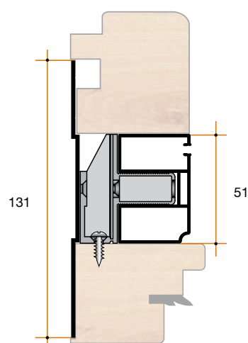
Esempio con compensatore alto.
