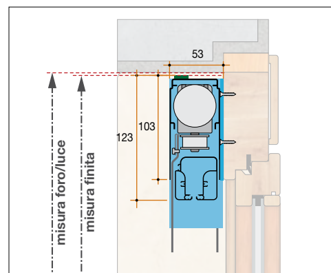
Sezione verticale 2 battenti con staffa attacco frontale
