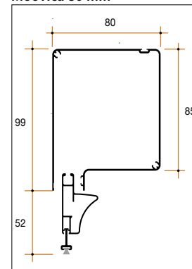
Ingombro gruppo Cassonetto Moovica 80 mm
