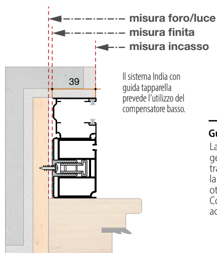
Esempio di installazione Guida Tapparella da 90 mm
