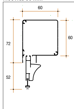
Ingombro gruppo Cassonetto Moovica 60 mm
