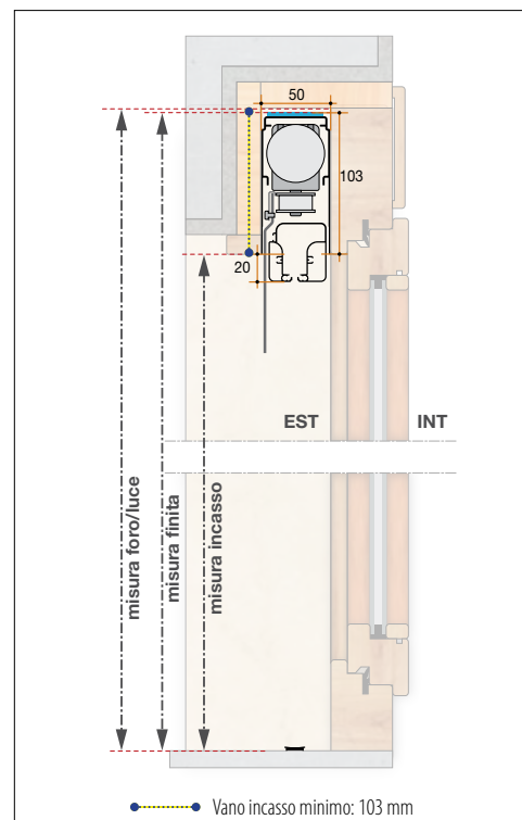
Sezione verticale 2 battenti con staffa attacco superiore
