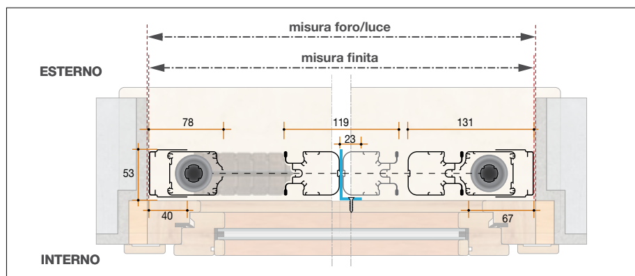
Sezione orizzontale 2 battenti con staffa attacco frontale
