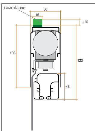
Ingombro carter e guida
