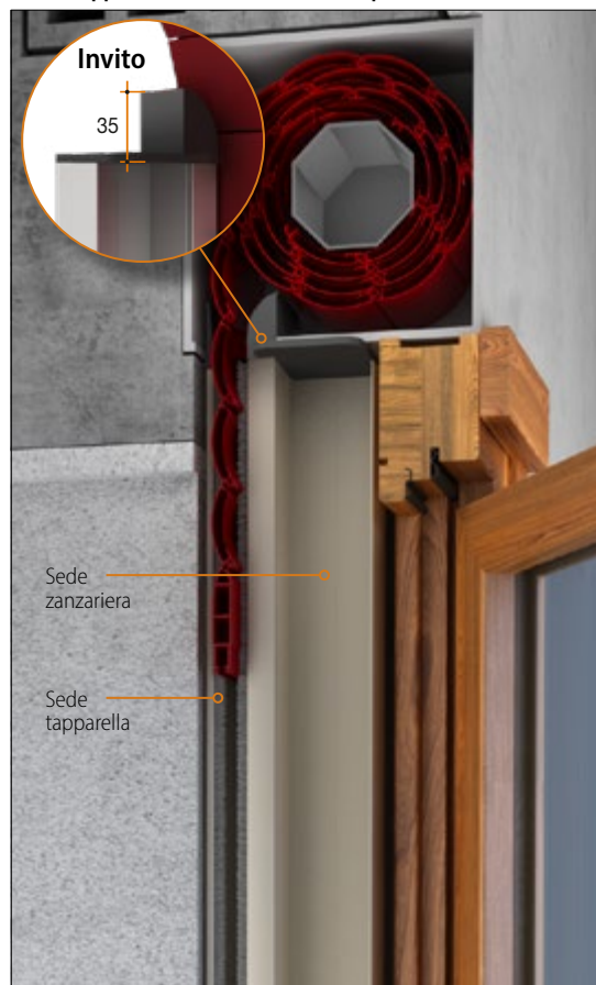
Esempio di installazione Guida Tapparella da 90 mm e compensatore basso
