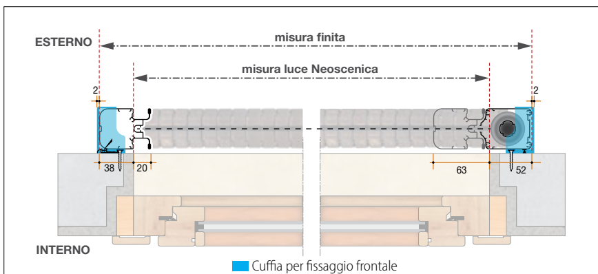
Sezione orizzontale 2 battenti
