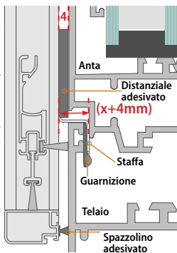
Serramento complanare
