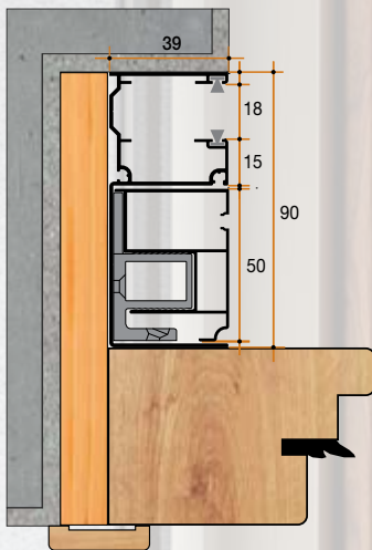
Esempio guida tapparella da 90 mm con guida e compensatore modello Delta
