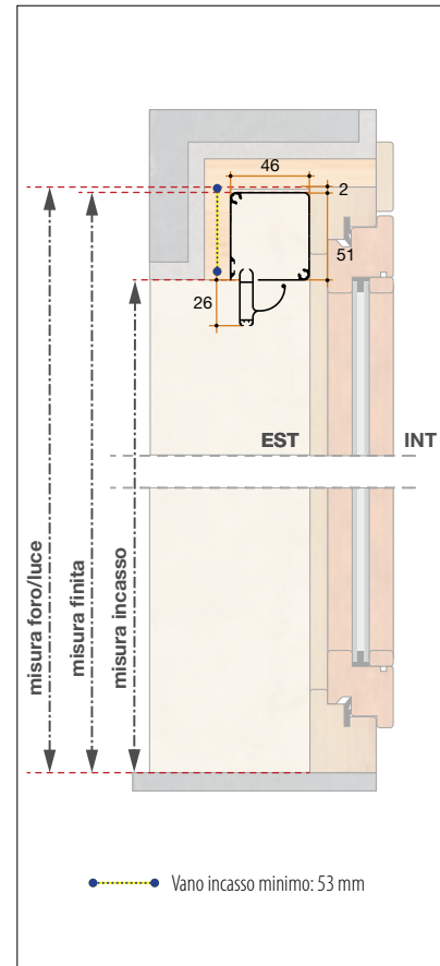
Sezione verticale
