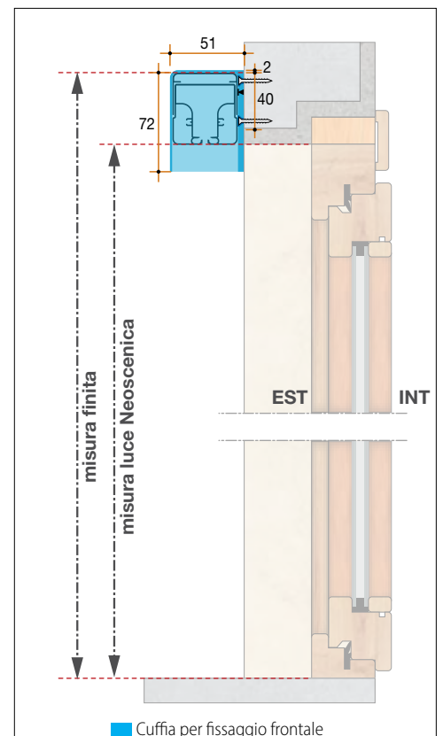
Sezione verticale
