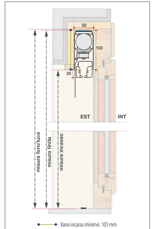
Sezione verticale 2 battenti con staffa attacco superiore
