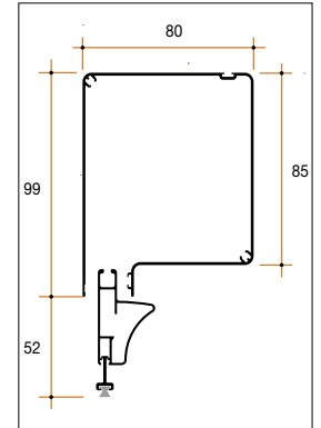
Ingombro gruppo Cassonetto Moovica 80 mm
