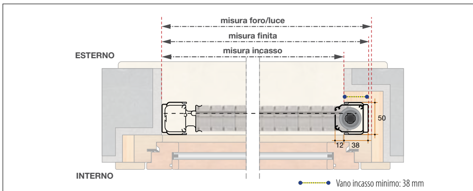
Sezione orizzontale con opzione "Incasto 2 lati".
