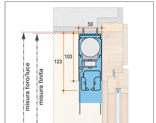
Sezione verticale 2 battenti con staffa attacco frontale
