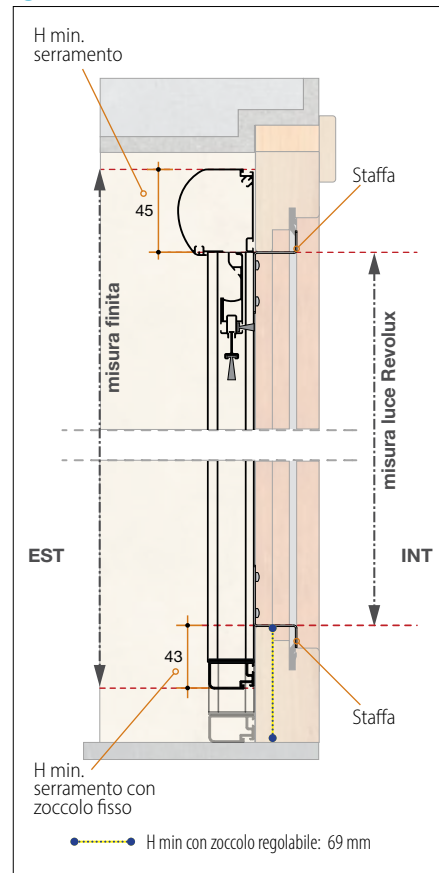
Serramento complanare
