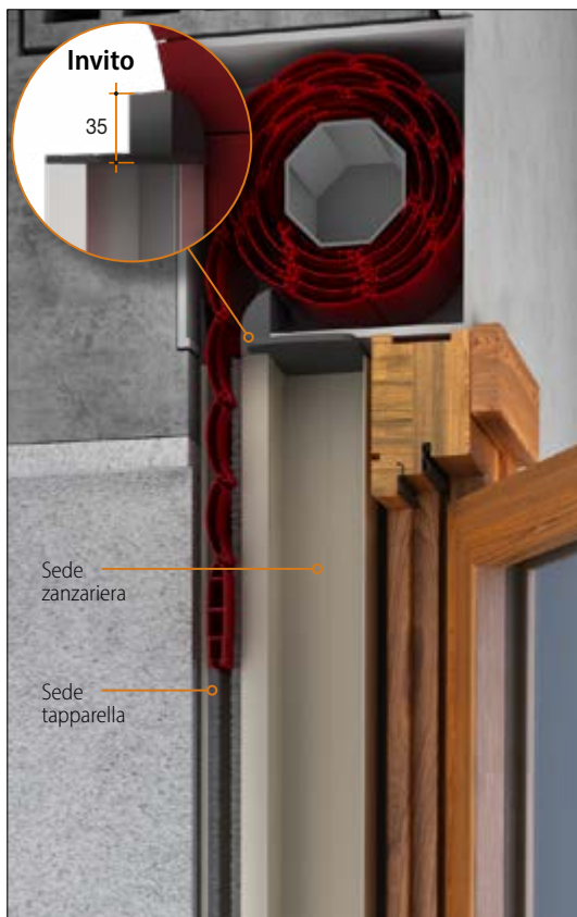
Esempio di installazione Guida Tapparella da 90 mm
