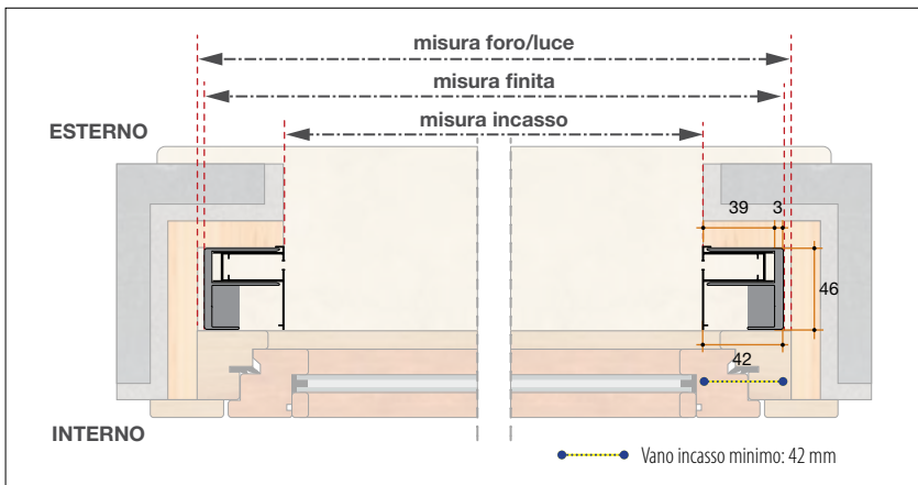
Sezione orizzontale
