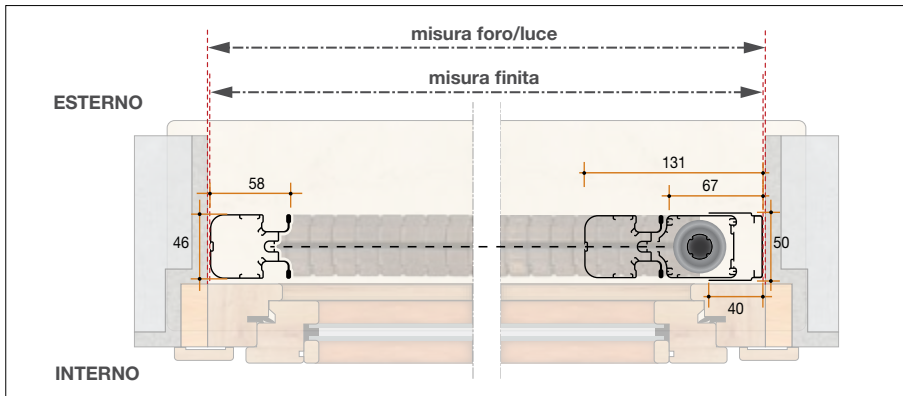
Sezione orizzontale 2 battenti con staffa attacco superiore
