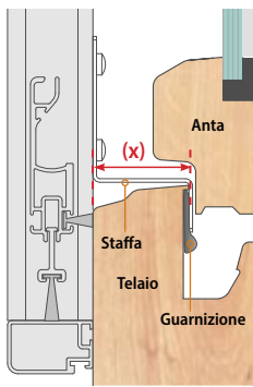
Serramento non complanare
