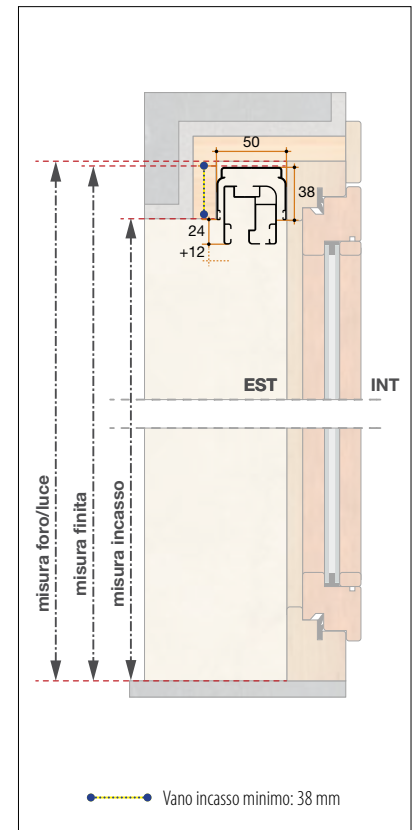
Sezione verticale
