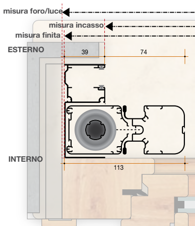
Esempio di installazione Guida Tapparella da 90 mm
