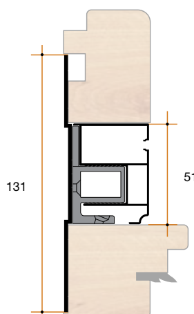
Esempio con guida e compensatore
