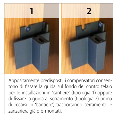
Tipologie di fissaggio
