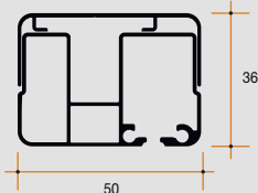
Guida telescopica Estetika® Motorizzata
