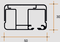
Guida telescopica Estetika®
