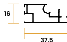
Copri tondino Rundstababdeckung
