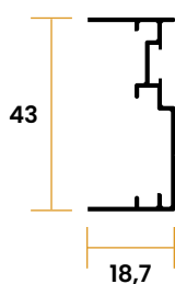
Compensatore a 2 vie 2-Wege-Ausgleichsprofil
