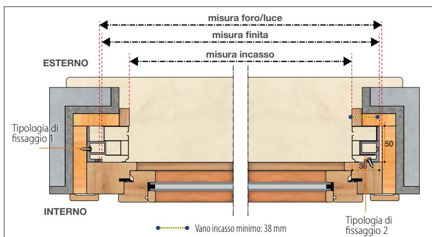
Sezione orizzontale
