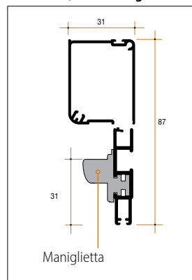
Cassonetto, barra maniglia
