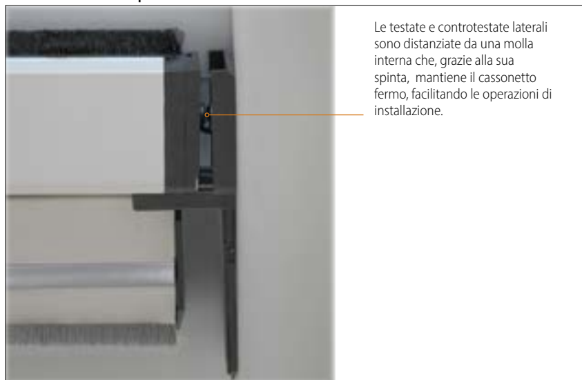
Testate con molla di espansione
