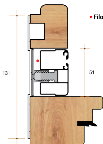
Esempio con guida e compensatore basso
