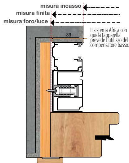
Esempio di installazione Guida Tapparella da 90 mm
