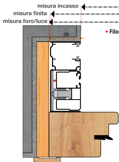
Esempio di installazione Guida Tapparella da 90 mm e compensatore basso
