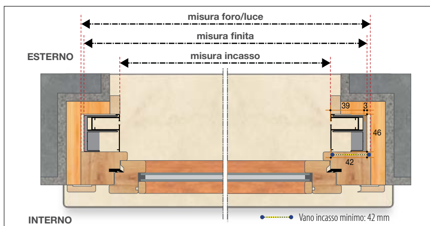
Sezione orizzontale
