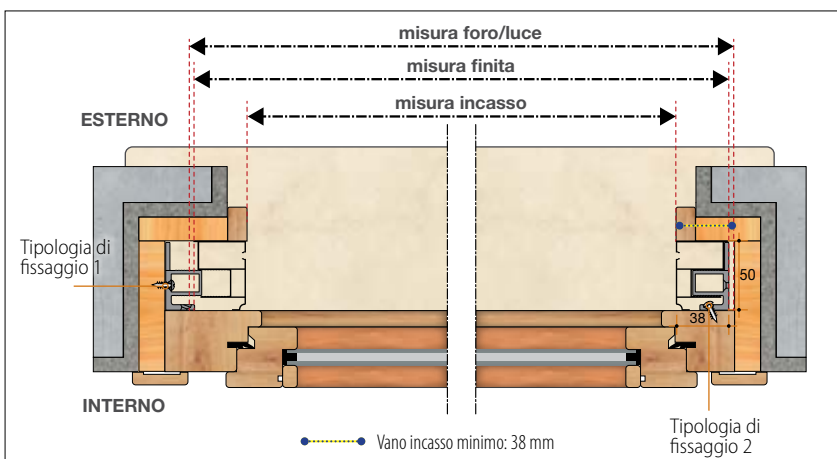
Sezione orizzontale
