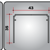
KIT 3213/.../B Profilo compensatore (L. 6000mm) Adjuster profile Profil adaptateur Ausgleichprofil Perfil adaptador
