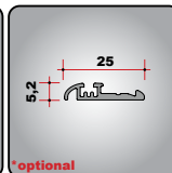
KIT 3214/..B Profilo di riscontro (L.5150mm) Side profile Profil lateral Seitlithprofil Perfil lateral
