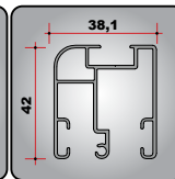
KIT 3312/... Guida (L. 6000mm) Track Coulisse Führungsschiene Gula
