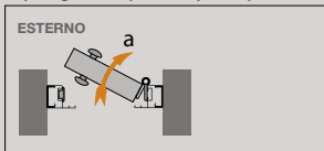
Tipologia A2 (1 anta apribile)
