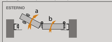
Tipologia A6 (2 ante apribili)
