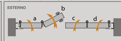
Tipologia A14 (4 ante apribili)
