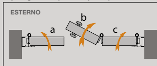
Tipologia A10 (3 ante apribili)
