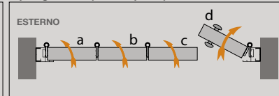
Tipologia A16 (4 ante apribili)
