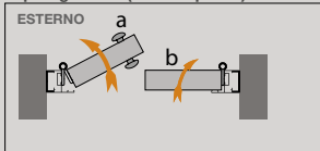
Tipologia A4 (2 ante apribili)
