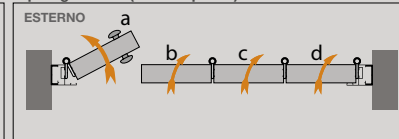
Tipologia A16 (4 ante apribili)
