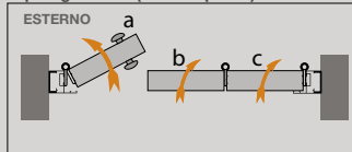
Tipologia A12 (3 ante apribili)
