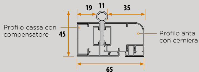
Tipologia A1 (1 anta apribile)
