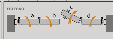
Tipologia A15 (4 ante apribili)
