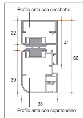
Tipologia A13 (4 ante apribili)
