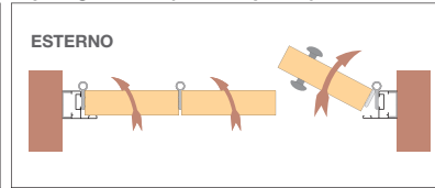
Tipologia A12 (3 ante apribili)
