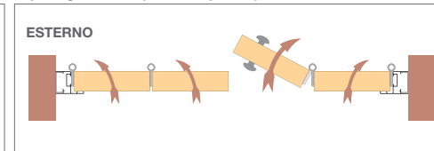
Tipologia A15 (4 ante apribili)
