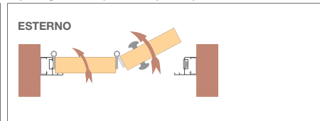
Tipologia A7 (3 ante apribili)
