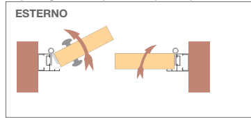
Tipologia A4 (2 ante apribili)
