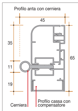
Tipologia A9 (3 ante apribili)
