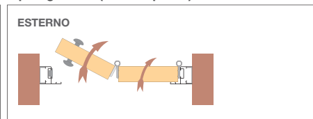
Tipologia A6 (2 ante apribili)
