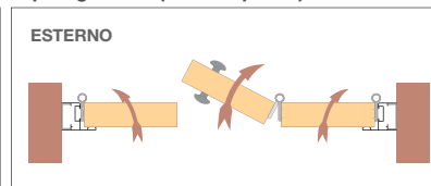
Tipologia A10 (3 ante apribili)
