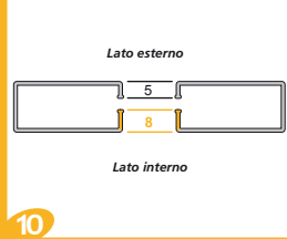
Inserire le guide Lato interno
