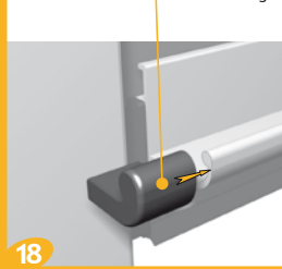
Inserire i PARASIGOLI alle estremità della barra maniglia
