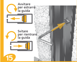
Con la chiave esagonale agire sui regolatori per ottimizzare la posizione delle guide
